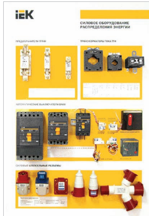
Силовое оборудование распределения энергии
