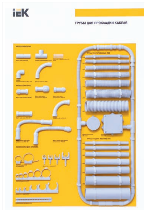
Трубы для прокладки кабеля
