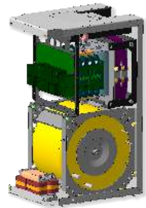
3-D модель стабилизатора «Каскад» серии 500
