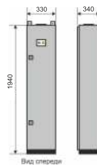
Габариты ИБП ФК
