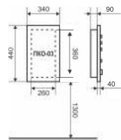
Посадочные размеры ПКО-03
