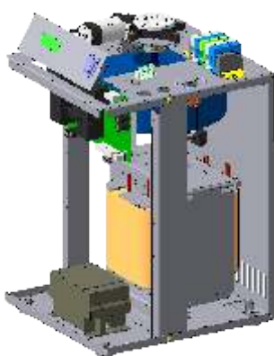
3-D модель стабилизатора «Сатурн» серии 500
